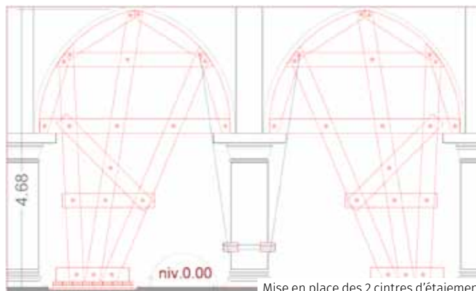
Mise en place des 2 cintres d'étalement
